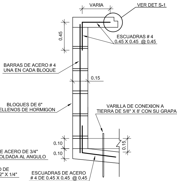
SECCION ESTRUCTURAL SIN ESCALA
