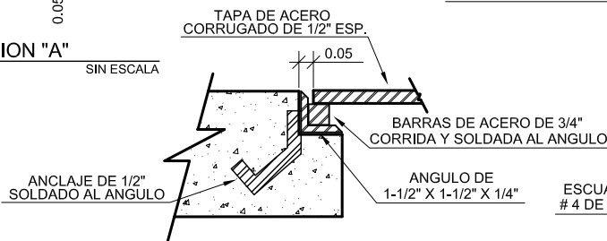
DETALLE S-1 SIN ESCALA
