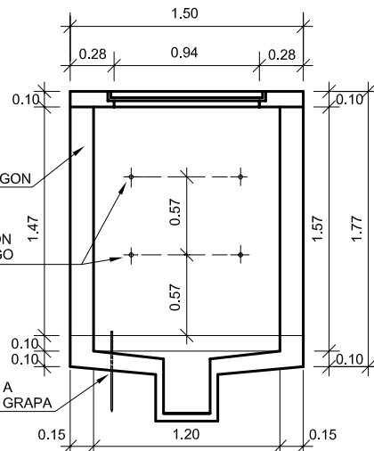
SECCION "B" SIN ESCALA
