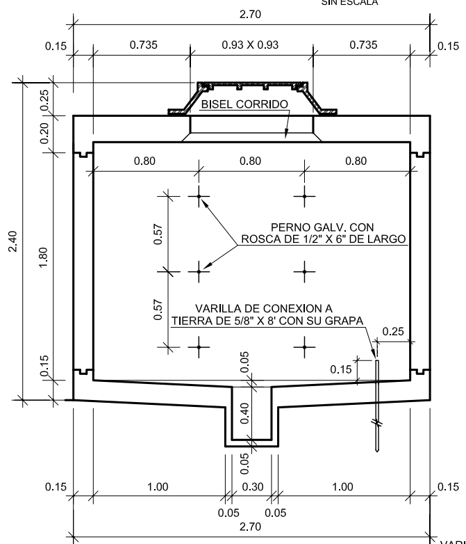
SECCION "A"
