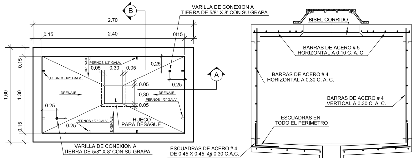
LOSA INFERIOR (PLANTA)
