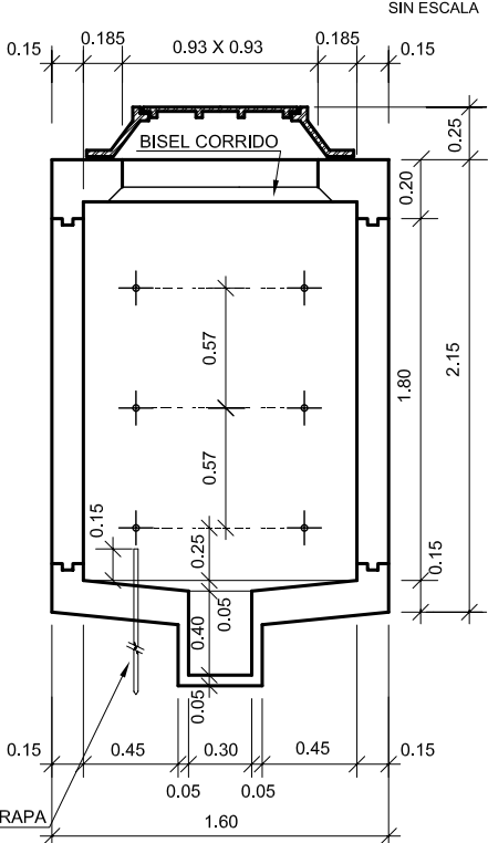
SECCION "B"
