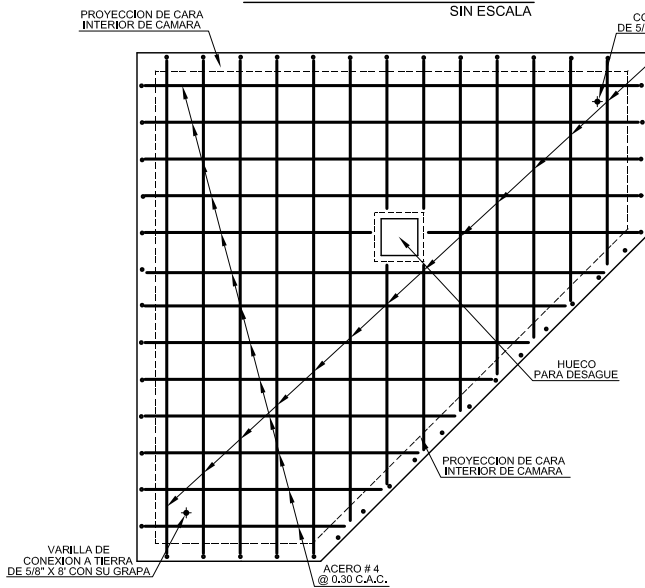
LOSA INFERIOR (PLANTA) SIN ESCALA
