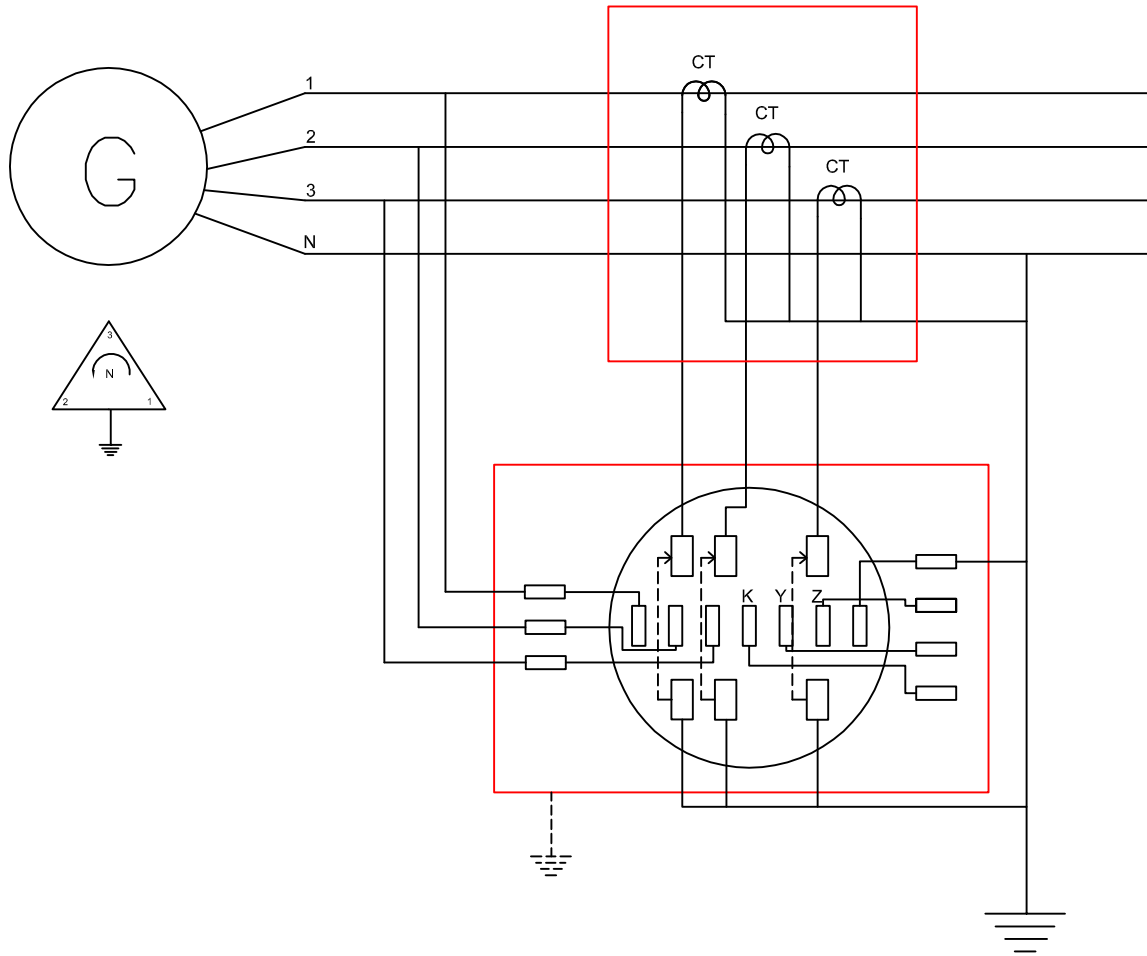
Conexión de medidor 9s, 3 fases, 4 hilos delta, 3 CT's
